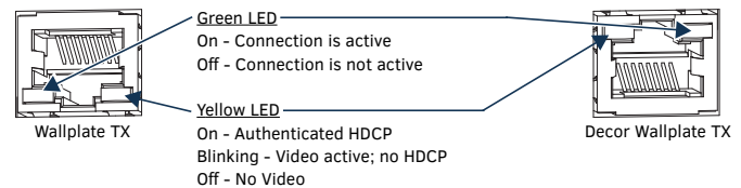
FIG. 6 DXLINK PORT LEDs
